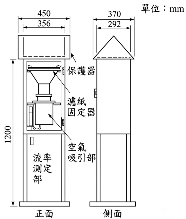
圖二 保護器之構造圖例
